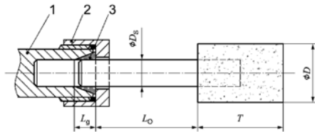
Εικόνα 1: Μήκος τοποθέτησης εργαλειοδέτη και κόλετ Υπόμνημα
