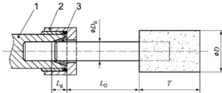
Bild 1: Einspannlänge von Spannfutter und Spannzanze
